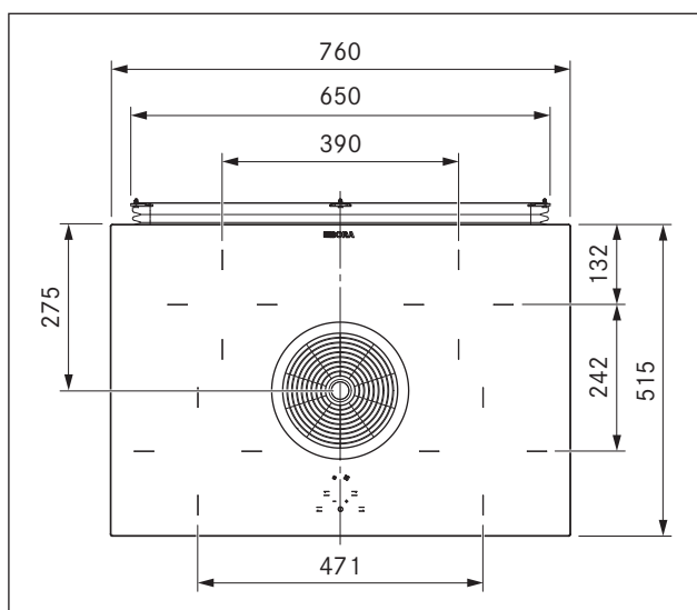
Prikaz 3.5 BIU dimenzije uređaja, prikaz odozgo
