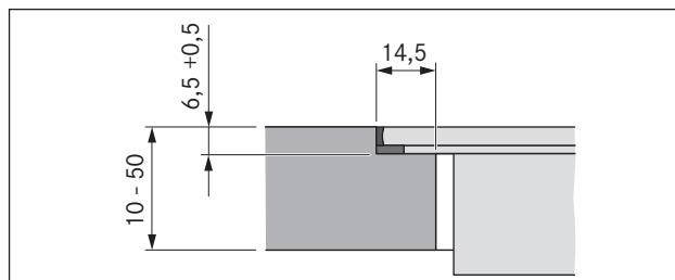
Prikaz 6.4 Dimenzije pregiba za montažu u ravlini s površinom
