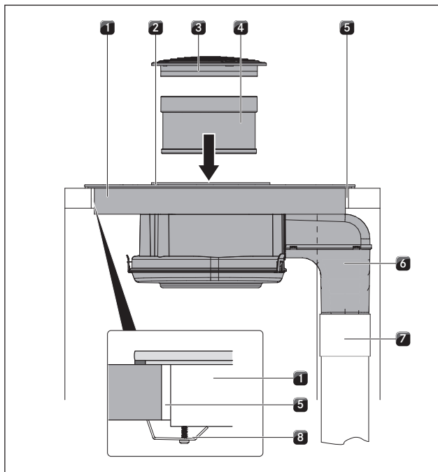
Prikaz 6.35 Priključivanje kanala za odvod zraka + učvršćivanje
