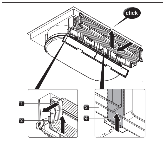
Prikaz 6.15 Vješanje okvira fleksibilnog kanala
