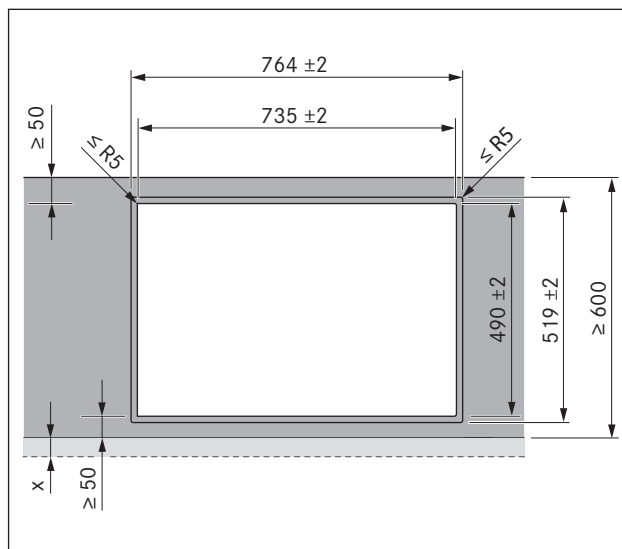
Prikaz 6.3 Dimenzije izreza za montažu u ravlini s površinom
