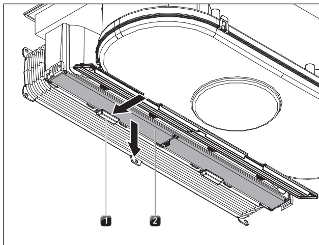
Prikaz 8.8 Uklanjanje filtra s aktivnim ugljenom
